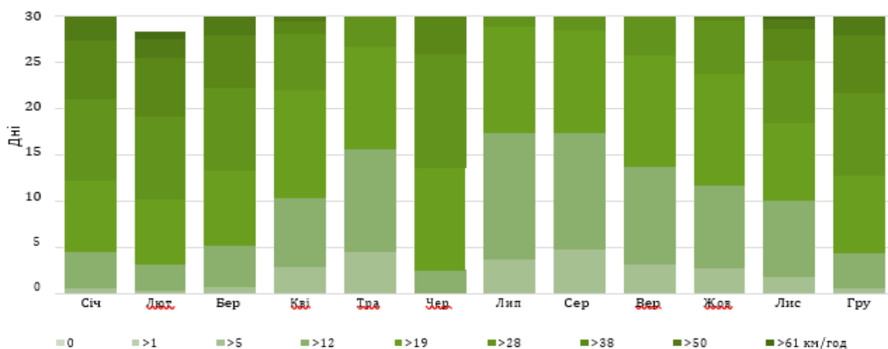
Рисунок. 00. Швидкість вітру
