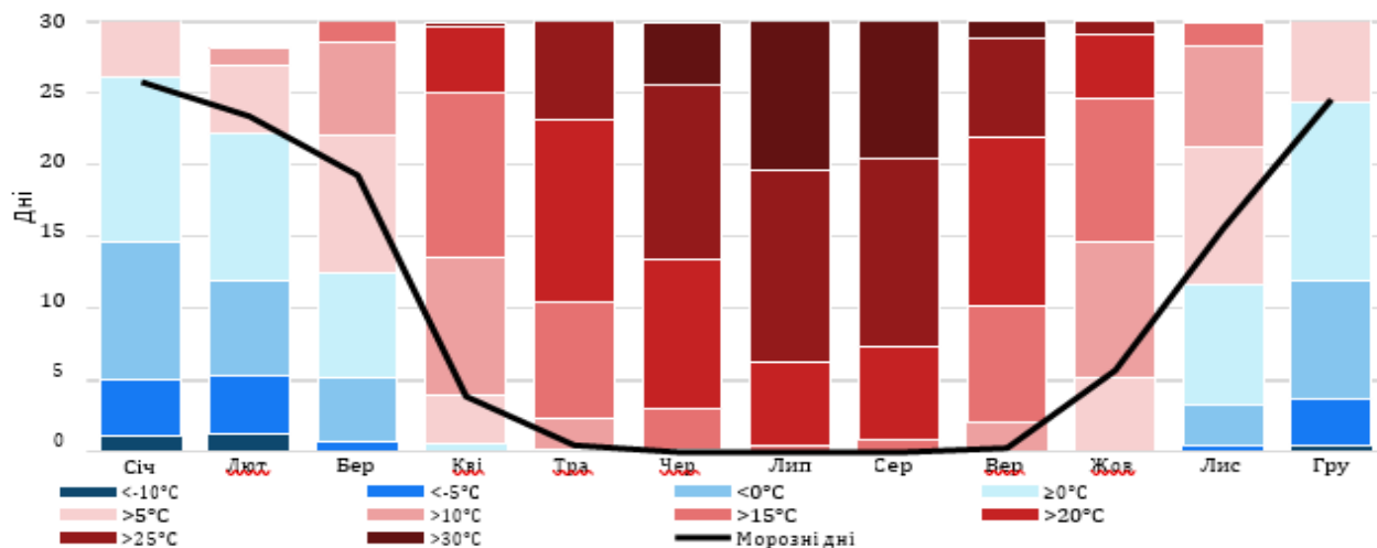
Рисунок. 00. Максимальні температури
